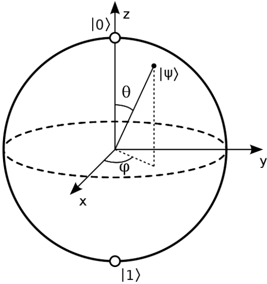
布洛赫球面呈現的量子位元
